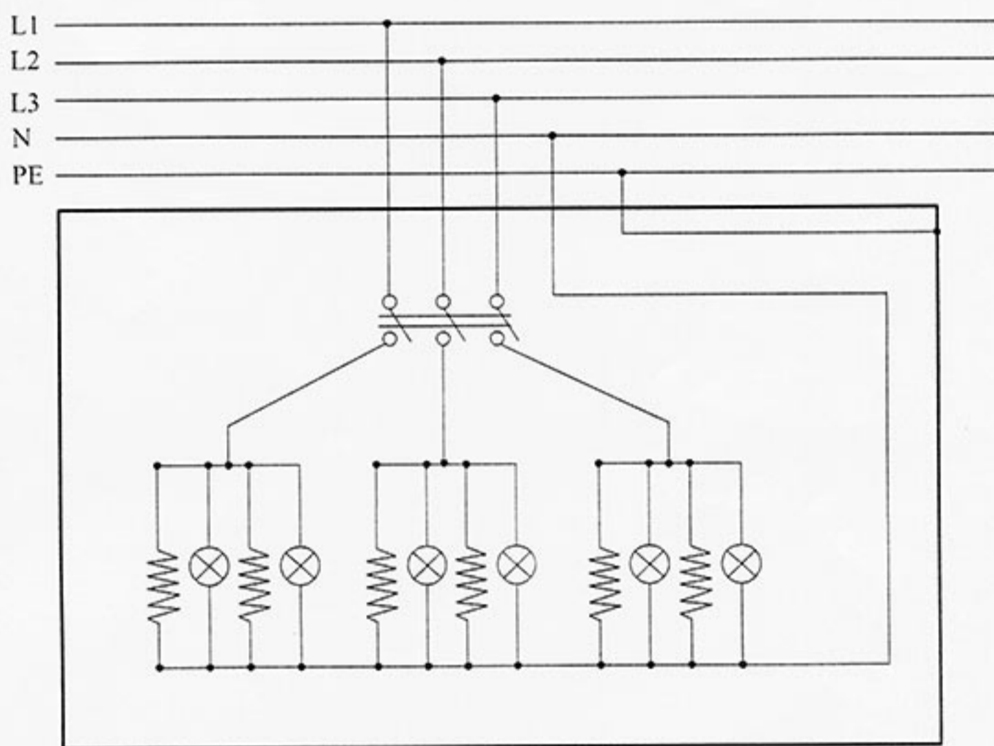
Električna šema
