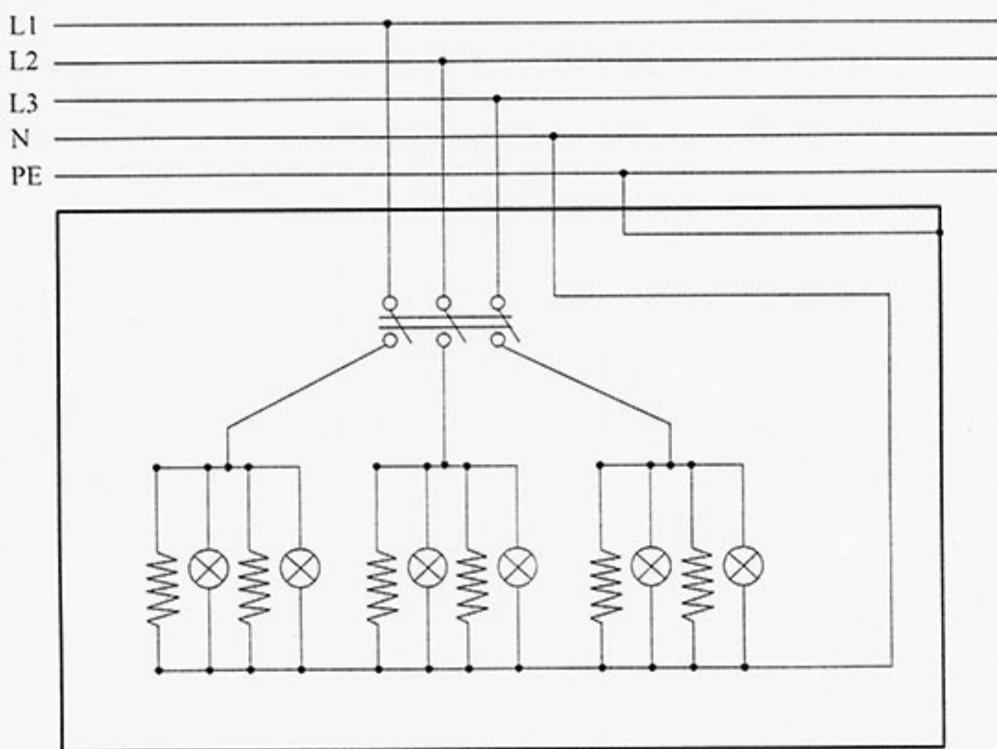
Električna šema
